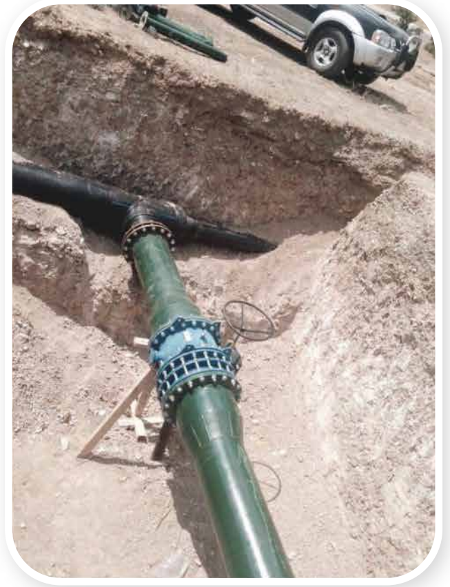
DENİZLİ - DARIVEREN GÖLETİ SULAMASI SANAT YAPISI - DERİN YAPILAR İMALAT ve MONTAJI
